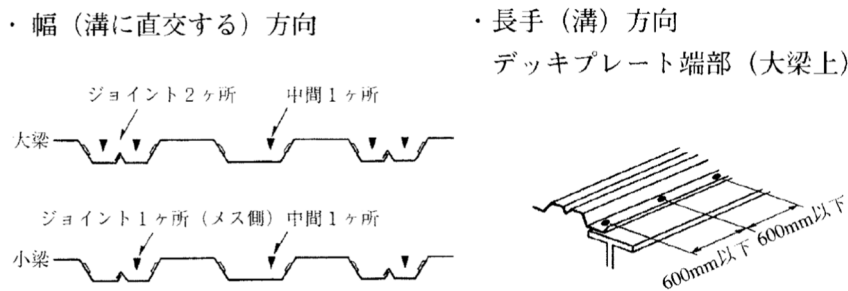
図 1 焼抜き栓溶接施工箇所
